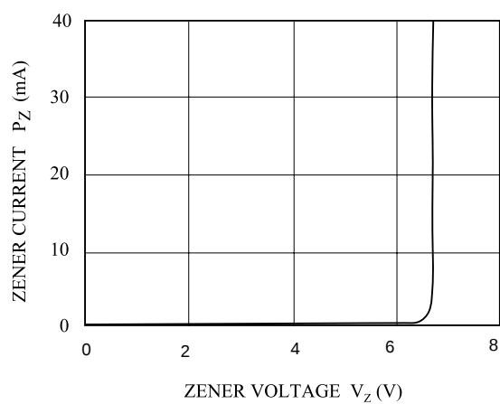
V_Z - I_Z
